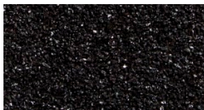
Karbíd křemíku
